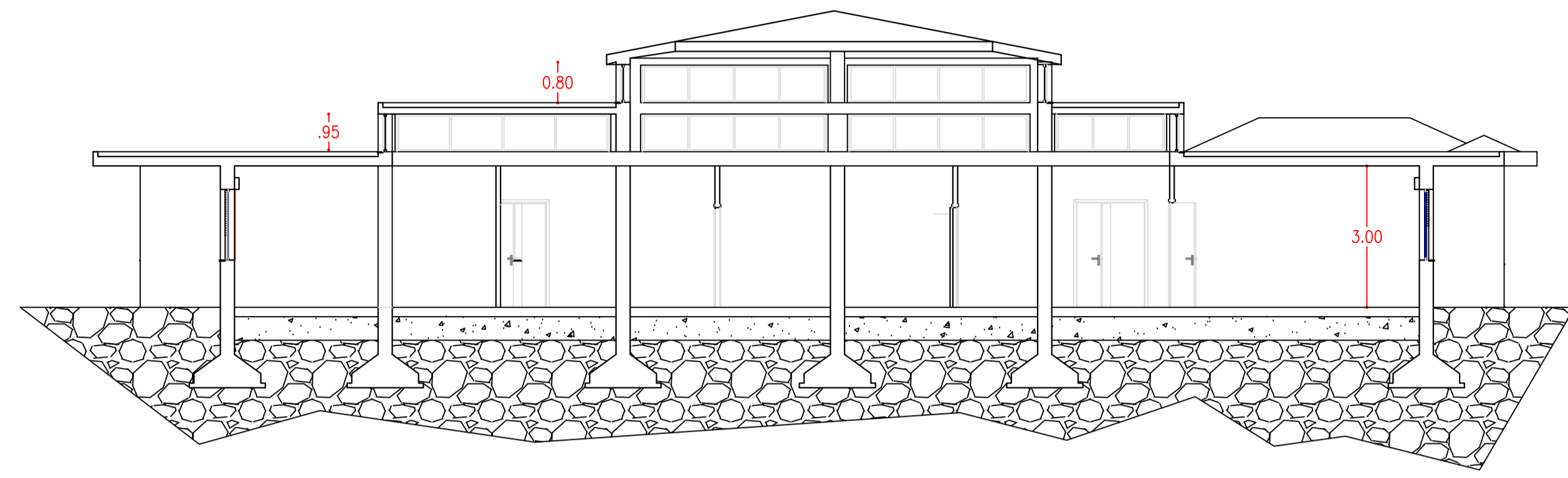
SEZIONE A-A
