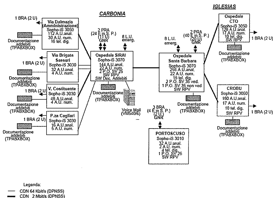
Figura 1 - Architettura Rete di Fonia
